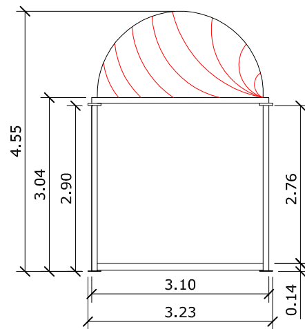
- PROSPETTO LATO 3 m
