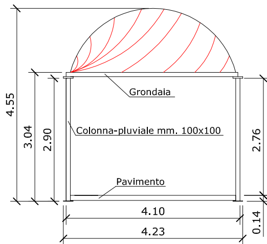
- PROSPETTO LATO 4 m
