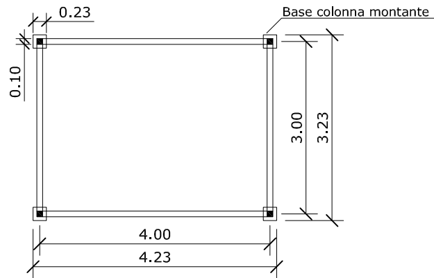
- PIANTA
