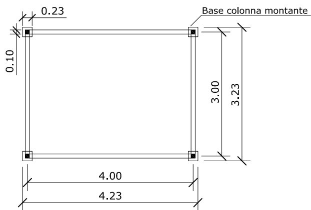
- PIANTA
