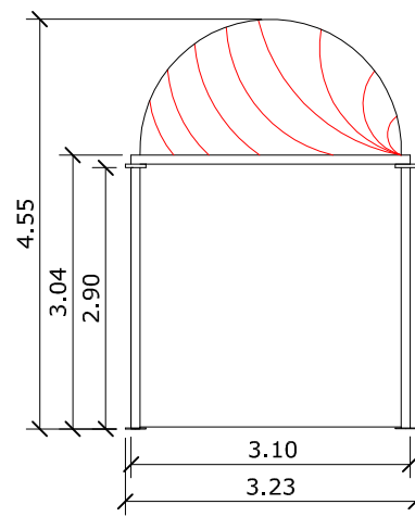
- PROSPETTO LATO 3 m
