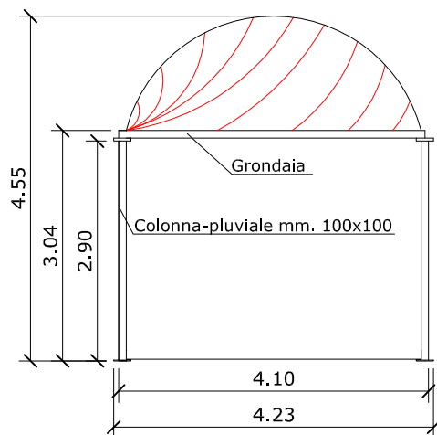
- PROSPETTO LATO 4 m
