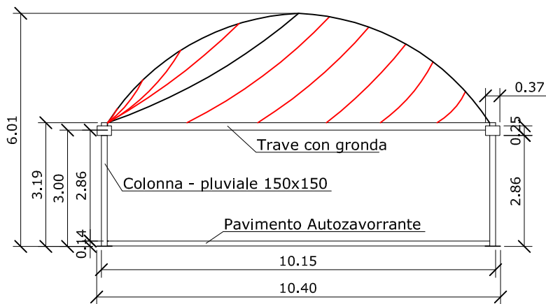
- PROSPETTO
