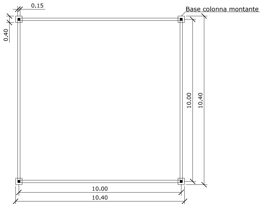
- PIANTA
