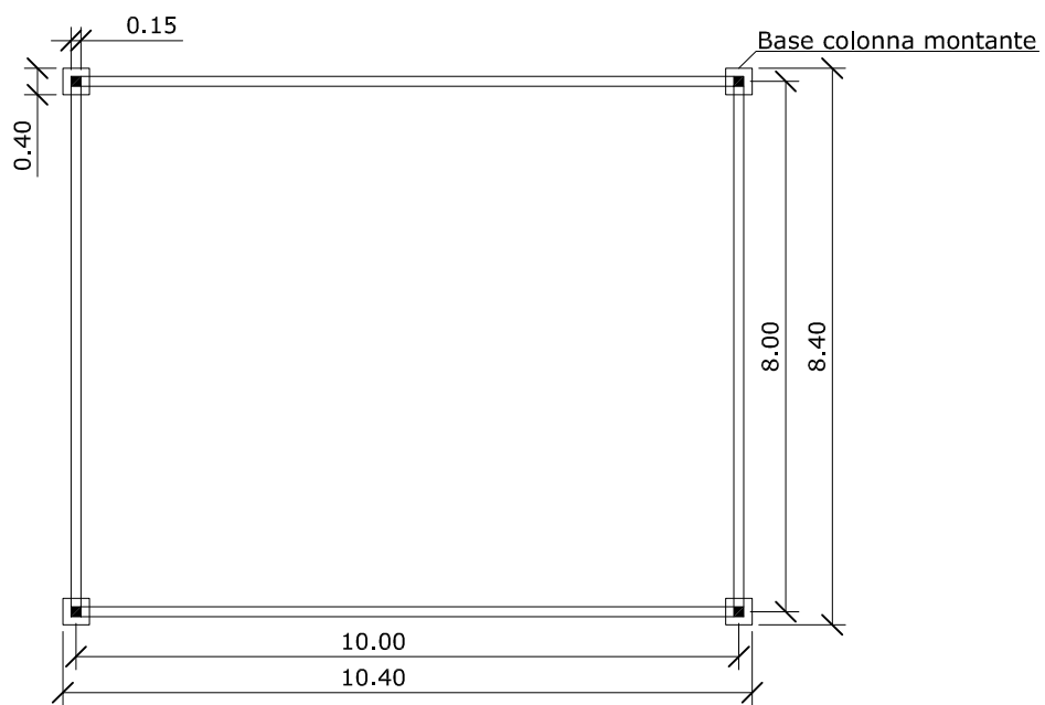
- PIANTA
