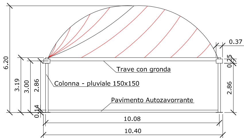
- PROSPETTO
