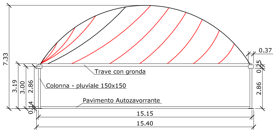
- PROSPETTO
