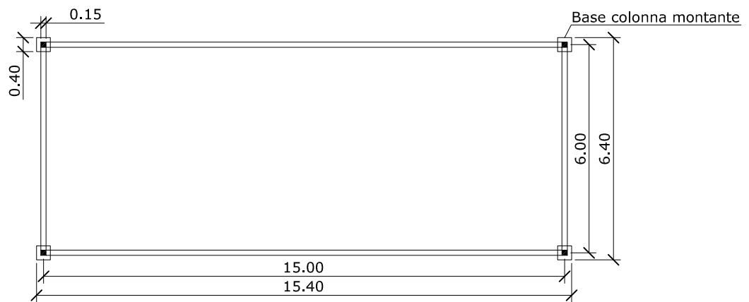
- PIANTA
