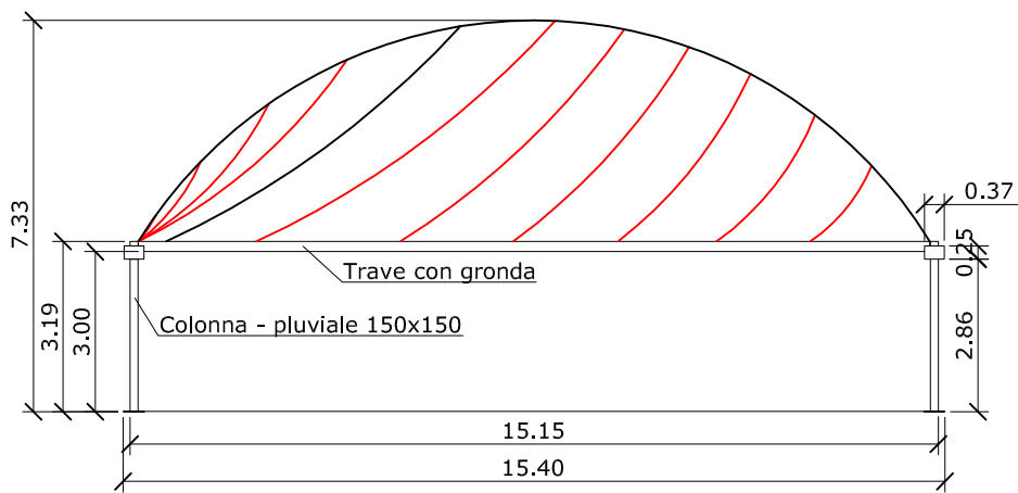
- PROSPETTO
