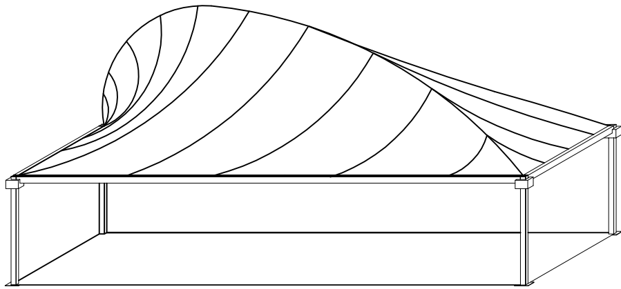
- ASSONOMETRIA
