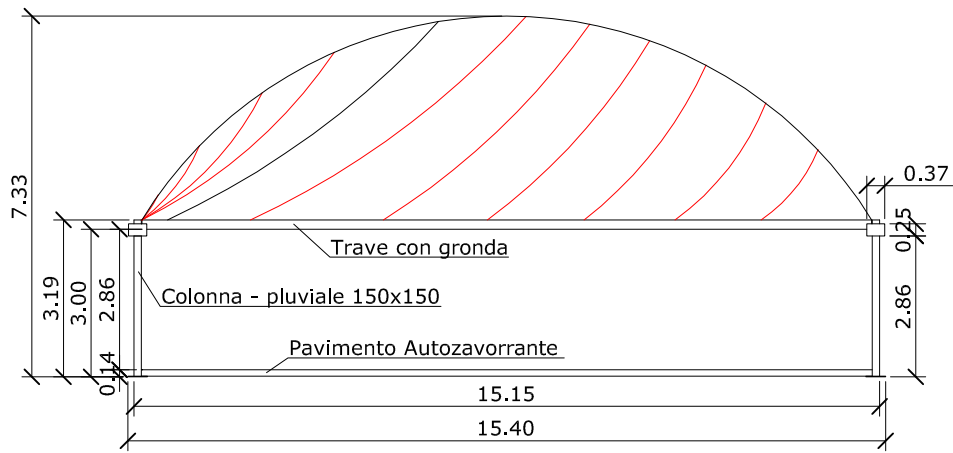
- PROSPETTO
