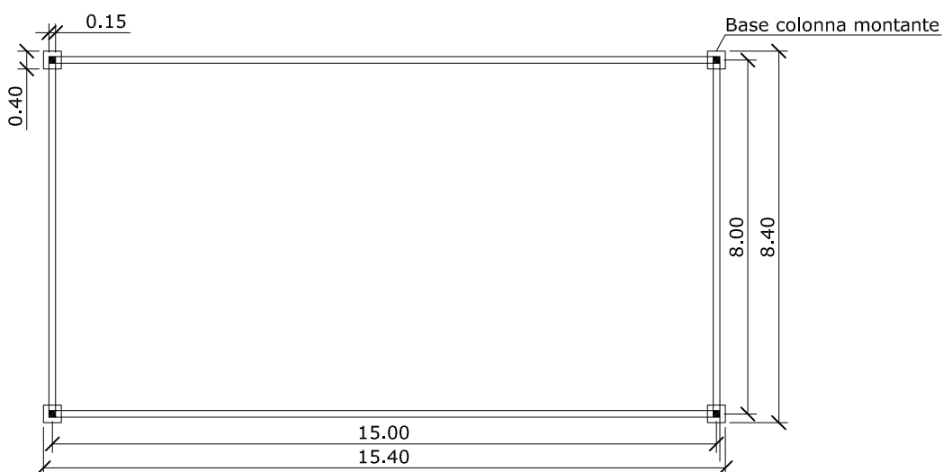
- PIANTA
