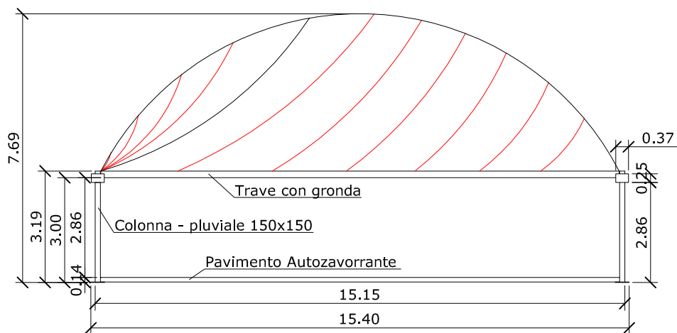
- PROSPETTO
