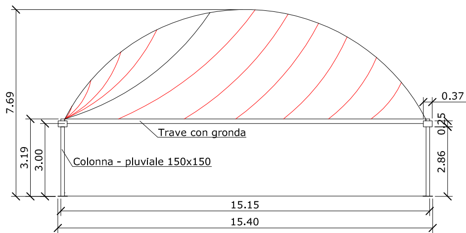
- PROSPETTO
