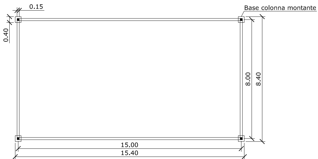
- PIANTA
