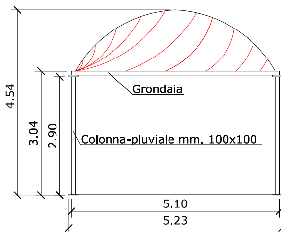
- PROSPETTO
