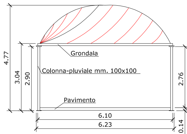
- PROSPETTO
