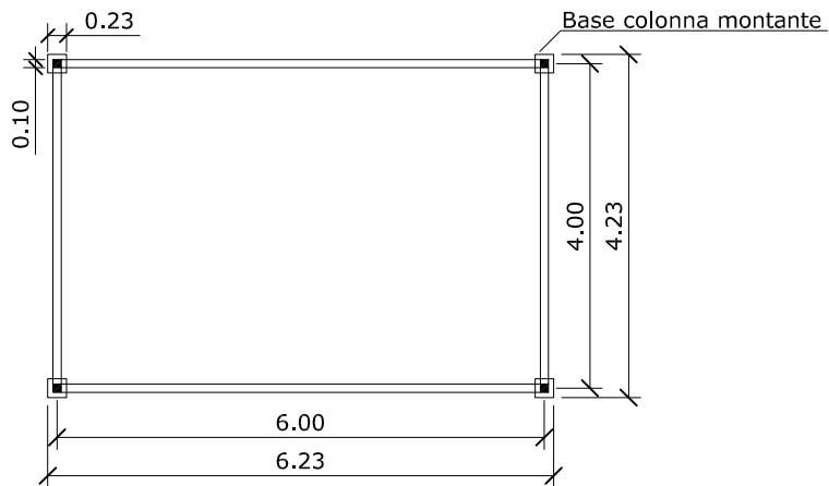
- PIANTA
