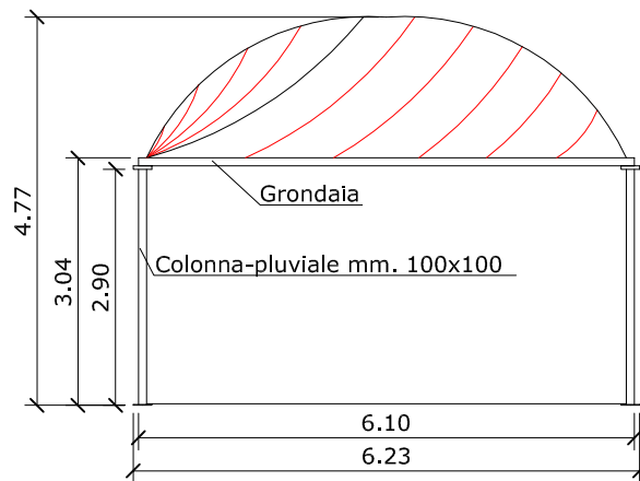
- PROSPETTO
