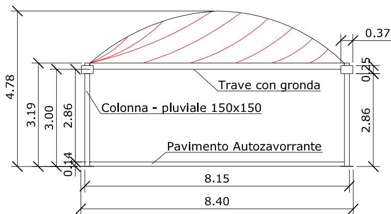
- PROSPETTO
