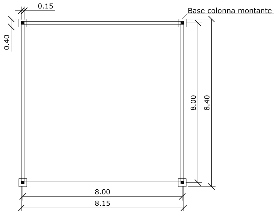
- PIANTA
