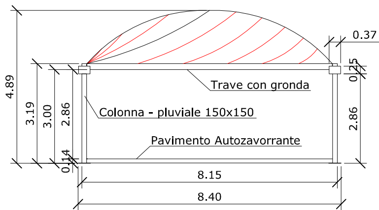
- PROSPETTO
