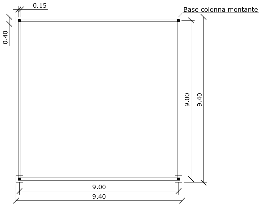
- PIANTA
