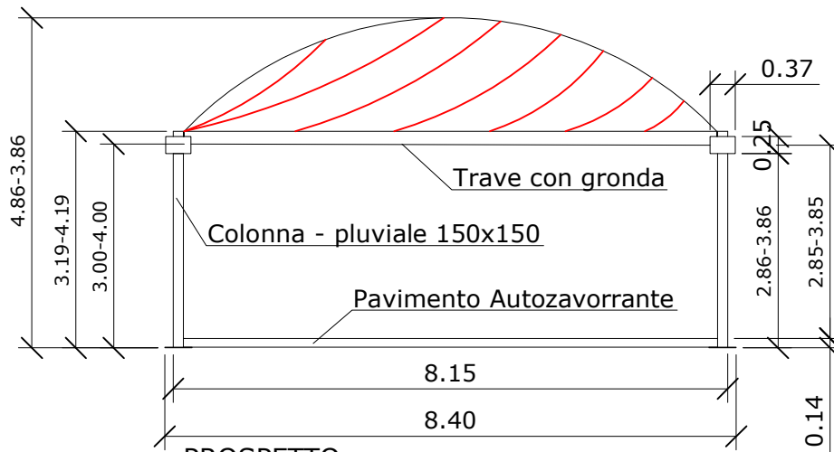
- PROSPETTO
