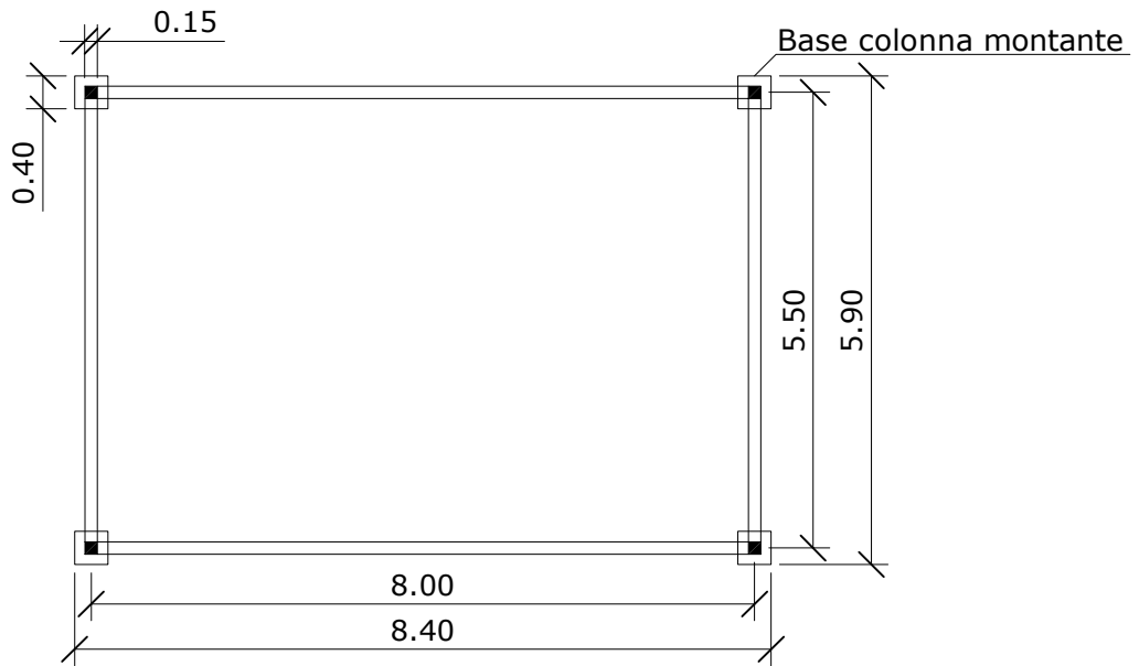
- PIANTA
