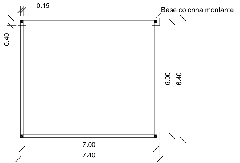
- PIANTA
