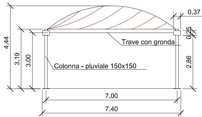
- PROSPETTO
