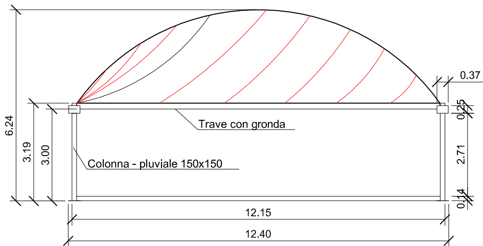
- PROSPETTO
