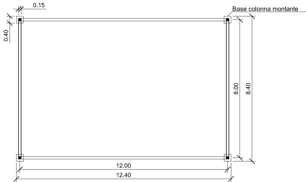
- PIANTA
