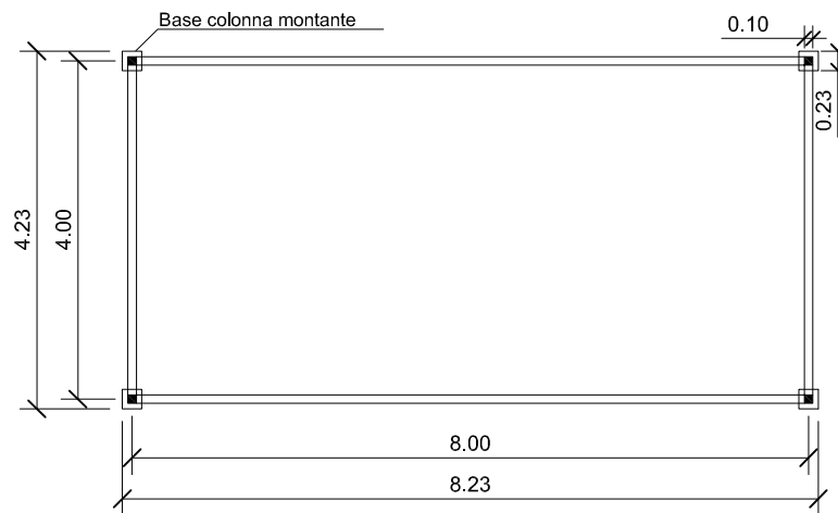
- PIANTA
