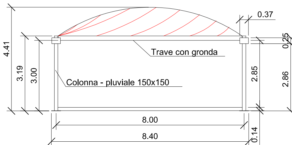
- PROSPETTO
