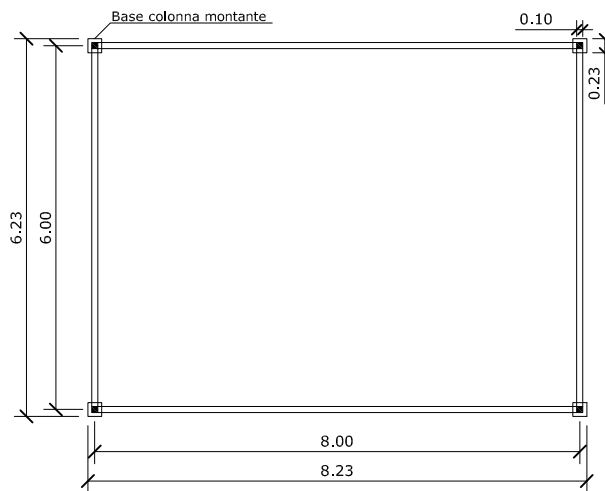
- PIANTA
