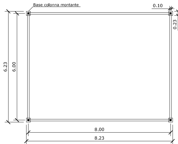
- PIANTA
