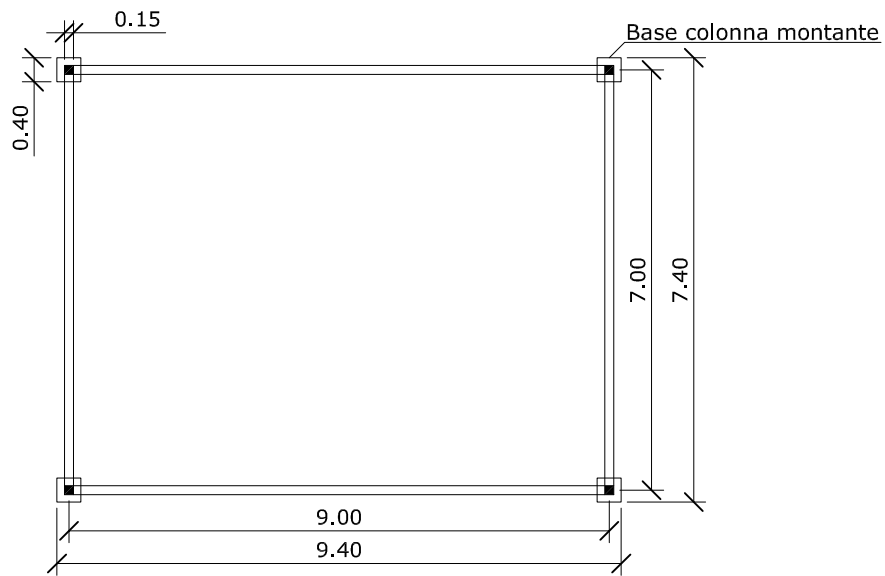
- PIANTA
