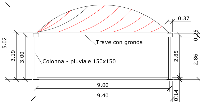
- PROSPETTO
