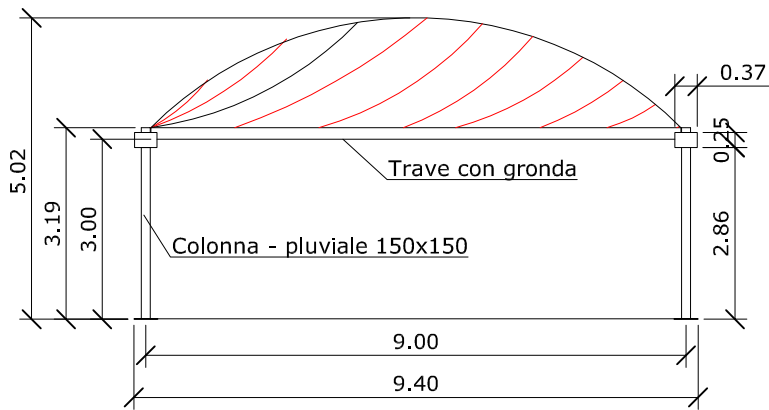
- PROSPETTO
