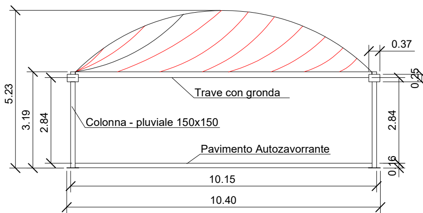
- PROSPETTO
