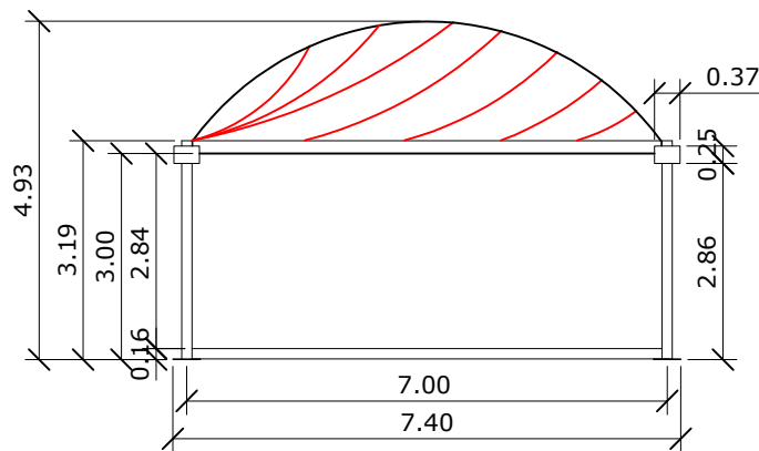
- PROSPETTO
