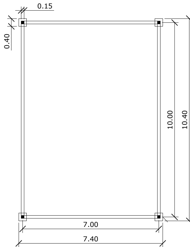
- PIANTA
