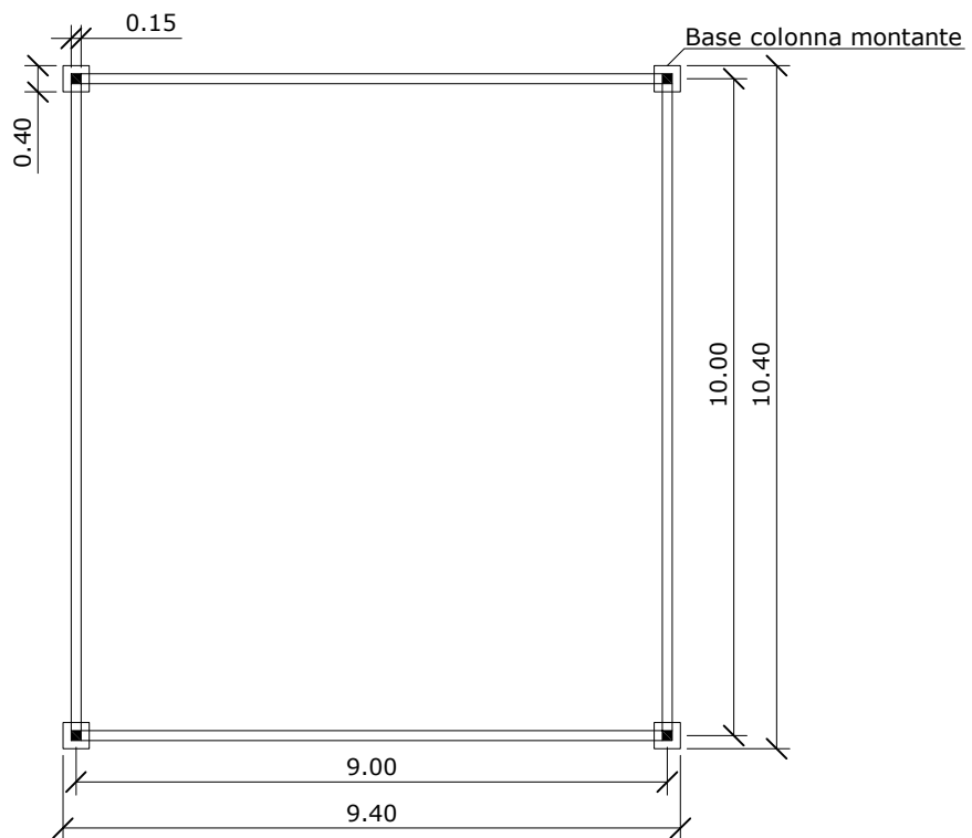
- PIANTA
