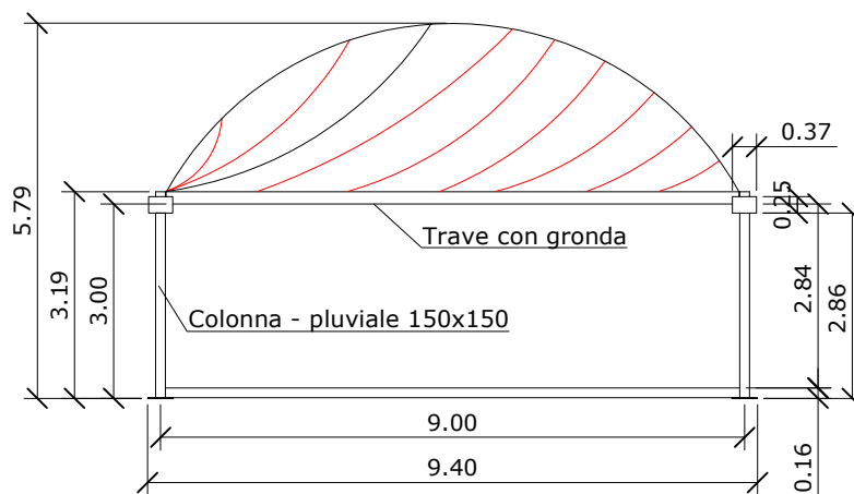
- PROSPETTO
