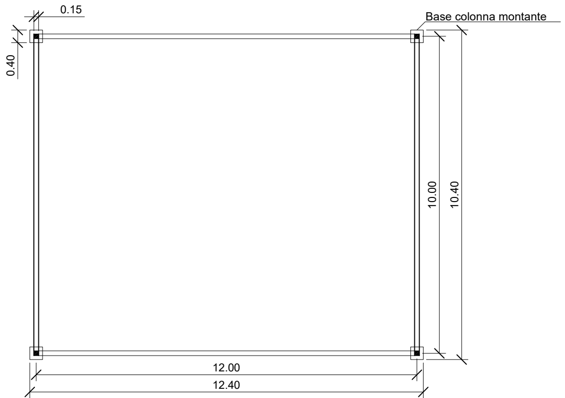
- PIANTA
