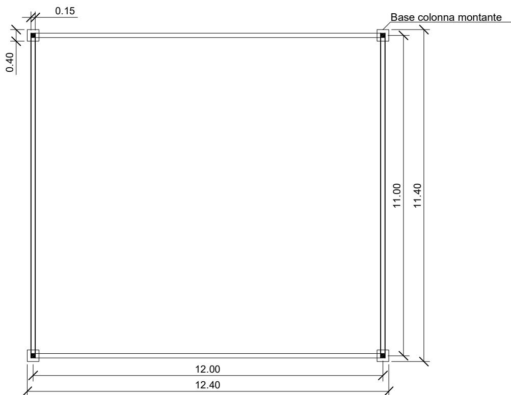
- PIANTA
