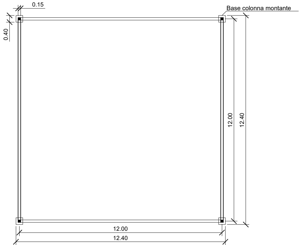
- PIANTA
