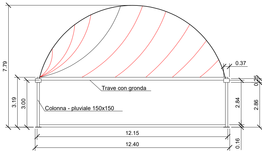
- PROSPETTO
