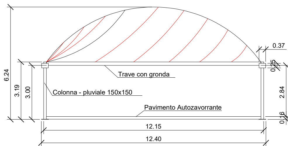
- PROSPETTO
