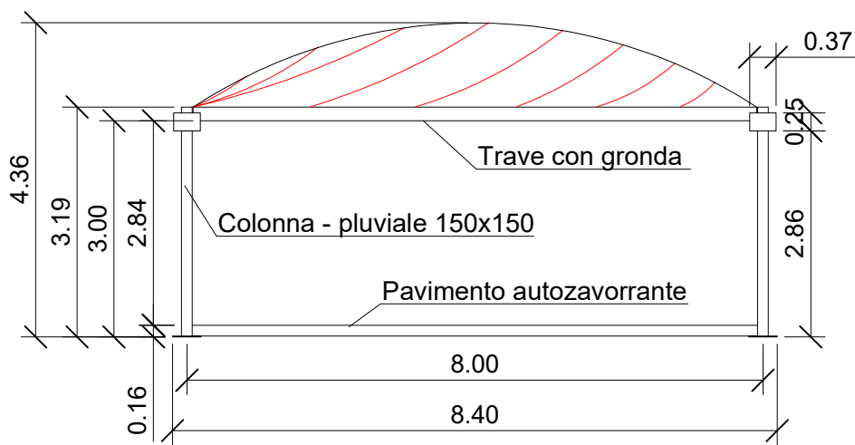
- PROSPETTO
