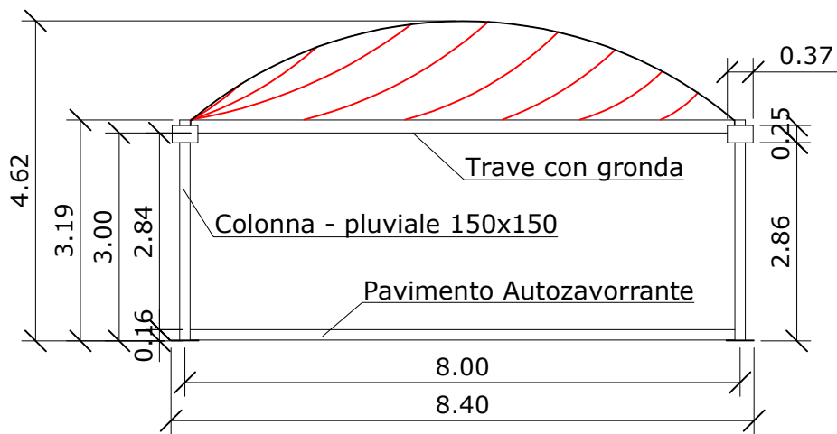
- PROSPETTO
