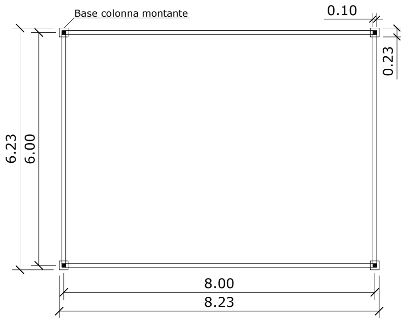
- PIANTA
