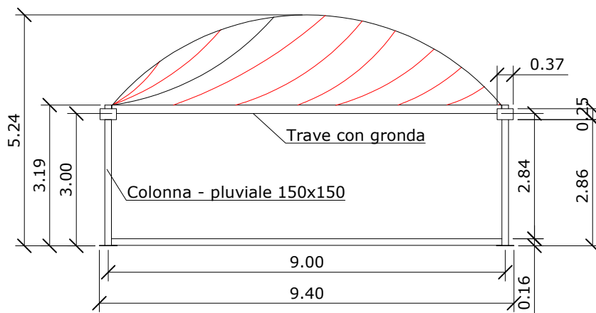
- PROSPETTO
