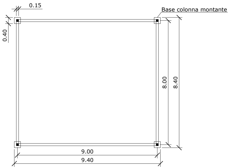
- PIANTA
