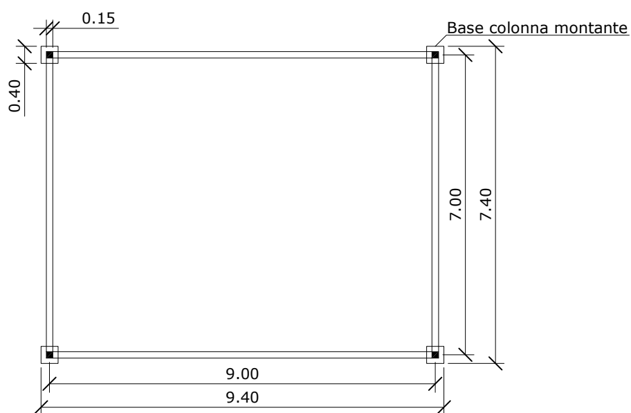
- PIANTA
