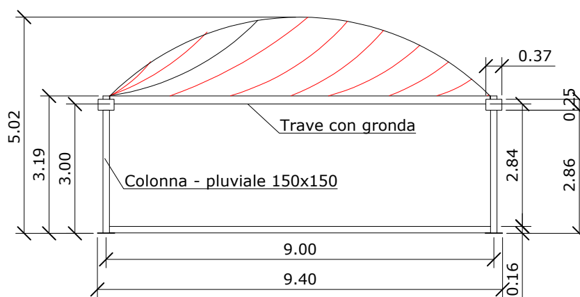
- PROSPETTO
