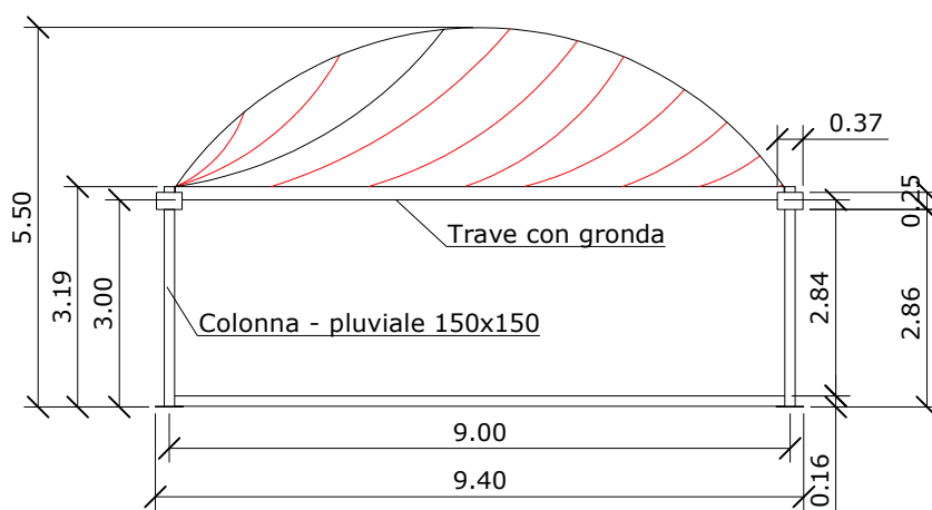
- PROSPETTO
