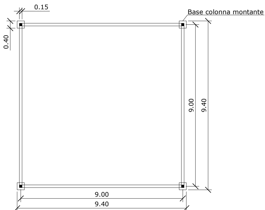
- PIANTA
